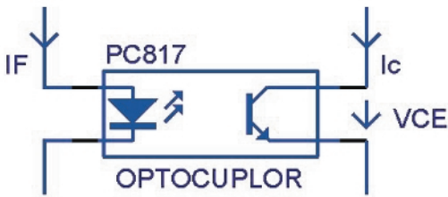
Fig. 2 Optocuplorul PC 817
