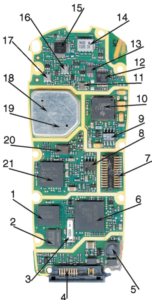
Fig. 1a Placa "SIM&Microcontroller" fața 1
