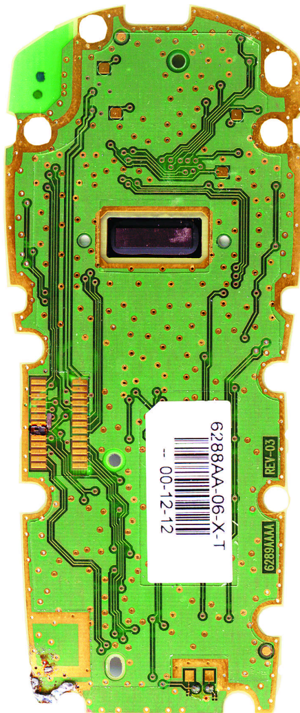
Fig. 1d Placa "LCD", fața 2
