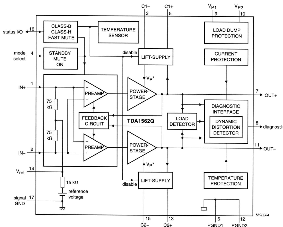
Fig. 1 Schema internă a circuitului TDA1562Q
