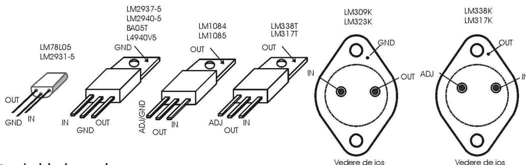
Fig. 5 Dispunerea terminalelor la capsule
