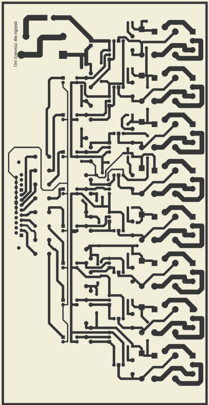
Fig. 4 Desenul cablajului imprimat
