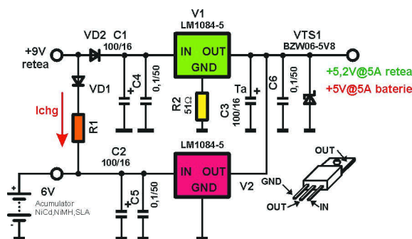
Fig. 12 Stabilizator cu ieșire mare în curent - 5A
