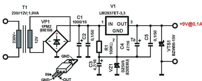
Fig. 8 Alimentator pentru aparat de măsură
