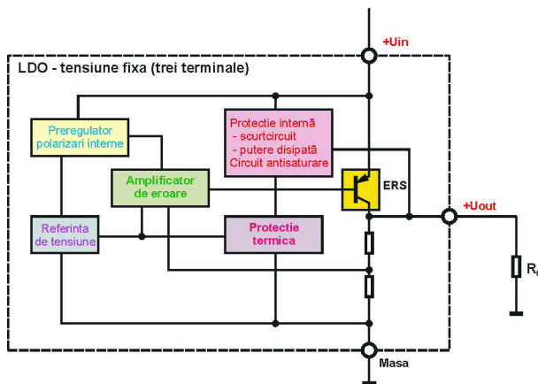
Fig. 3 Schema bloc a unui stabilizator LDO
