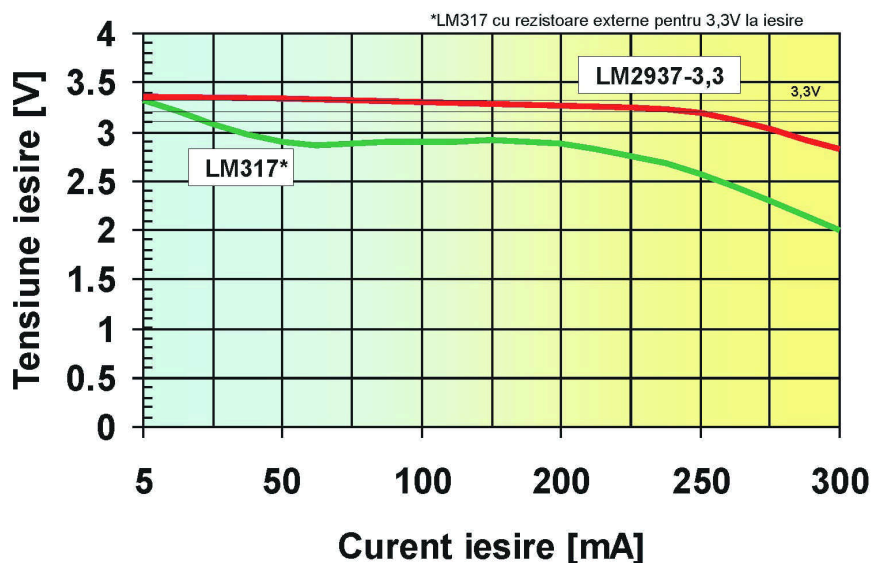
Fig. 11 Caracteristică U-I comparativă pentru stabilizatorul din figura 7
