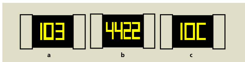
Fig. 4 Exemplu de marcare a rezistoarelor "chip" cu trei digiți (a), cu patru digiți (b), cu trei digiți conform EIA-96 (c)
