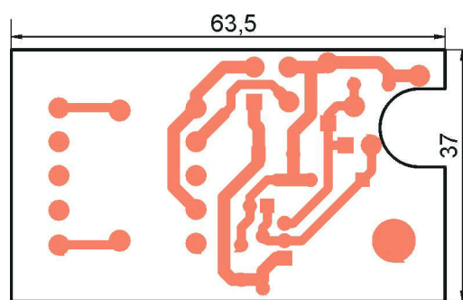
Fig. 9 Cablajul imprimat corespunzător satbilizatoarelor din figurile 7 și 8.
