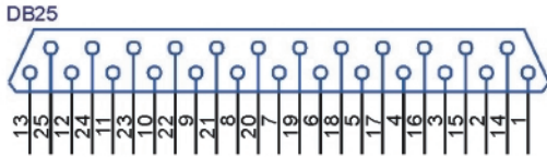
Fig.3 Conectorul portului paralel standard al calculatorului (PC)
