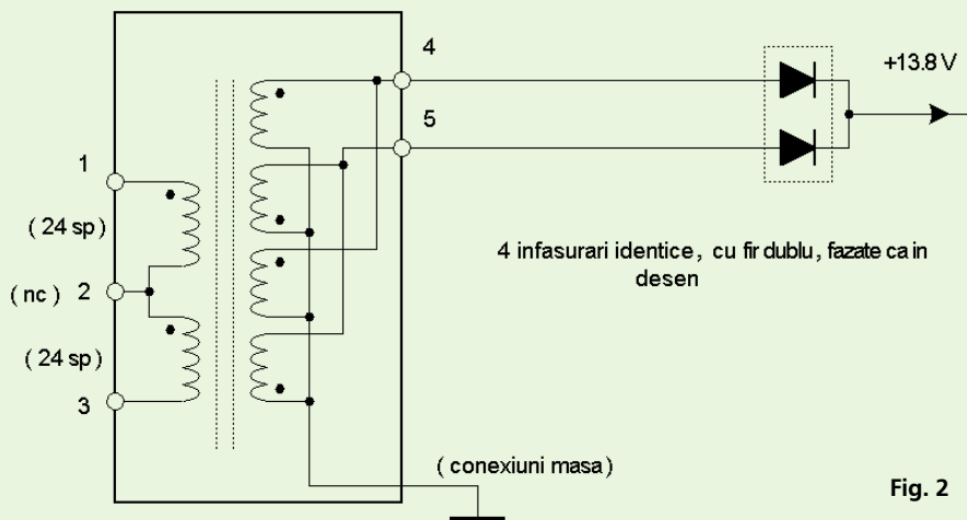
Trafo T1 in varianta proprie
