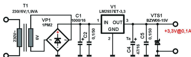
Fig. 7 Stabilizator de 3,3V alimentat de la rețea
