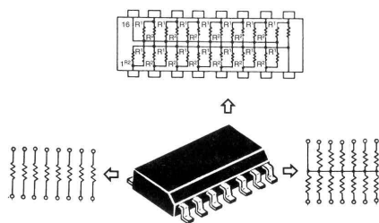
Fig. 6 Rețele rezistive SMD
