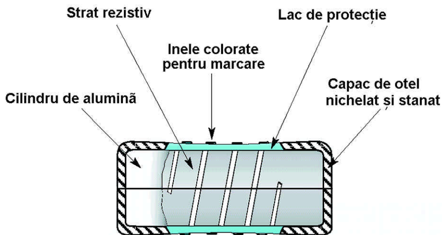
Fig. 5 Rezistoare MELF
